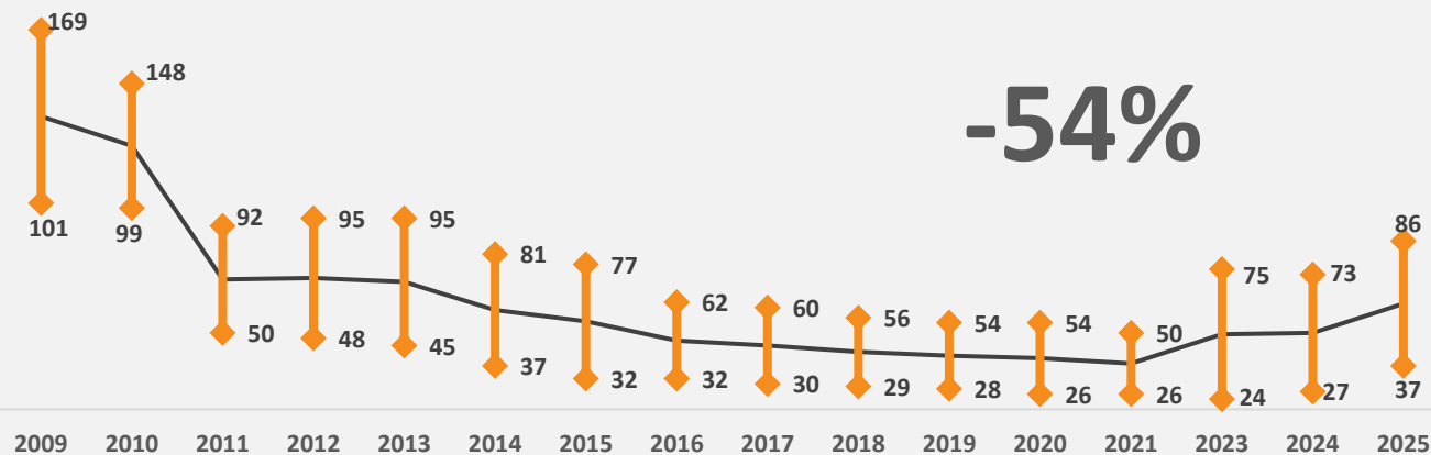
Custo de energia eólica não subsidiado ($/MWh)
