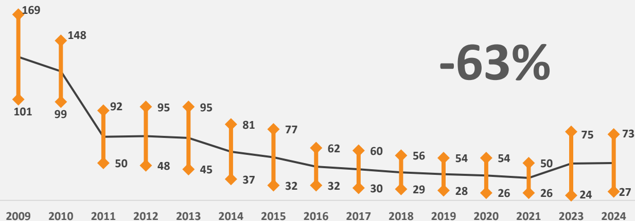
Custo de energia eólica não subsidiado ($/MWh)
